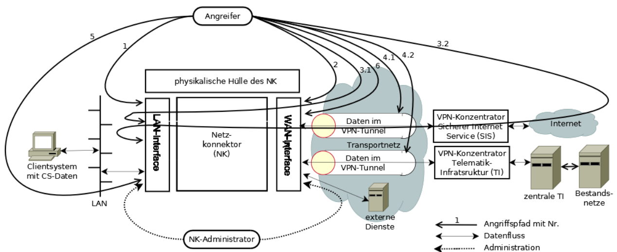
Abbildung 6: Externe Einheiten und Objekte im Zusammenhang, Angriffspfade
