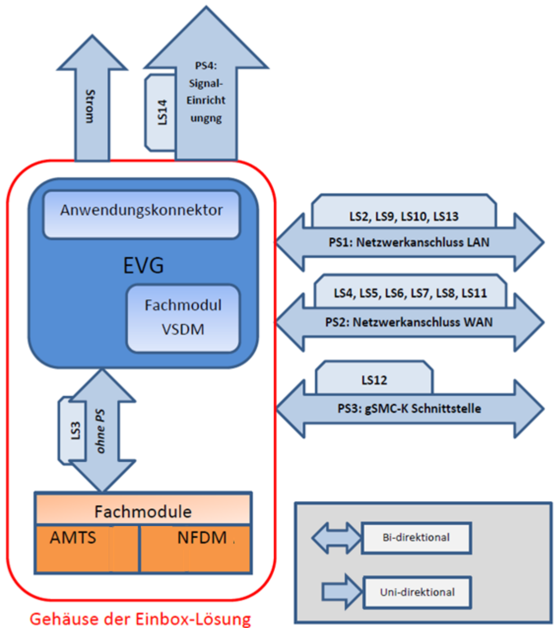
Abbildung 4: physische und logische externe Schnittstellen des Konnektors
