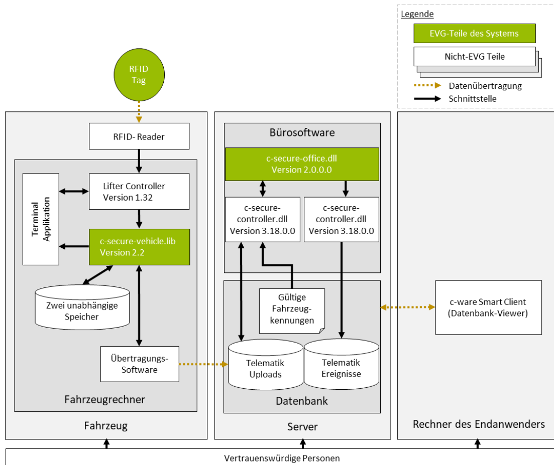
Abbildung 1: c-trace Abfall-Behälter-Identifikations-System c-ident
