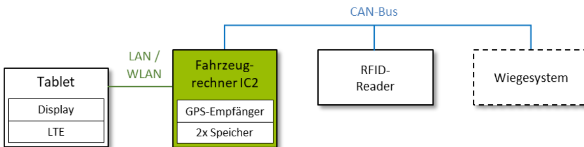
Abbildung 3: Fahrzeugsystem mit Fahrzeugrechner IC2
