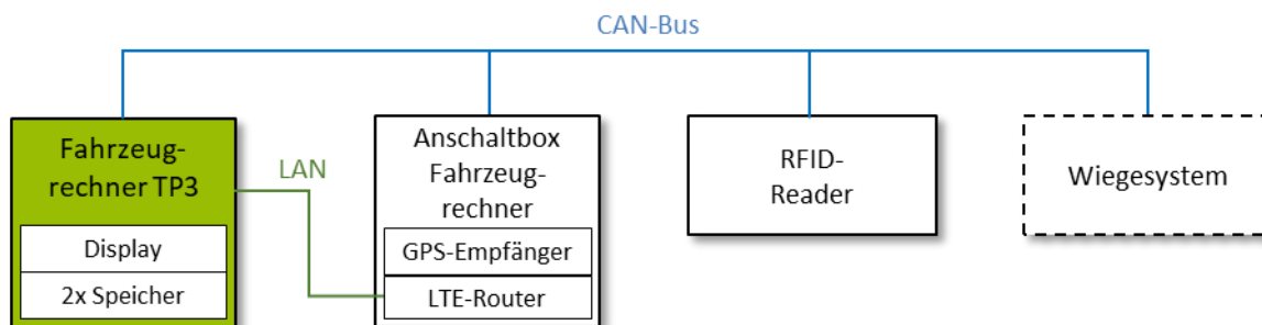
Abbildung 2: Fahrzeugsystem mit Fahrzeugrechner TP3
