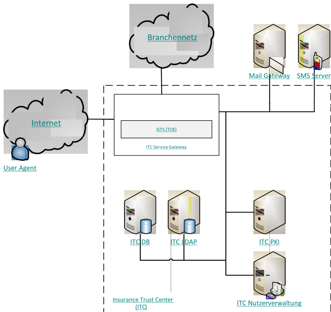
Abbildung 3 – ISTS Abgrenzung
