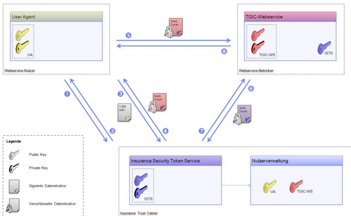
Abbildung 1 – ISTS Standardablauf
