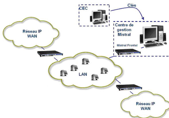
Figure 2 : Présentation du système Mistral (tunnel inversé)
