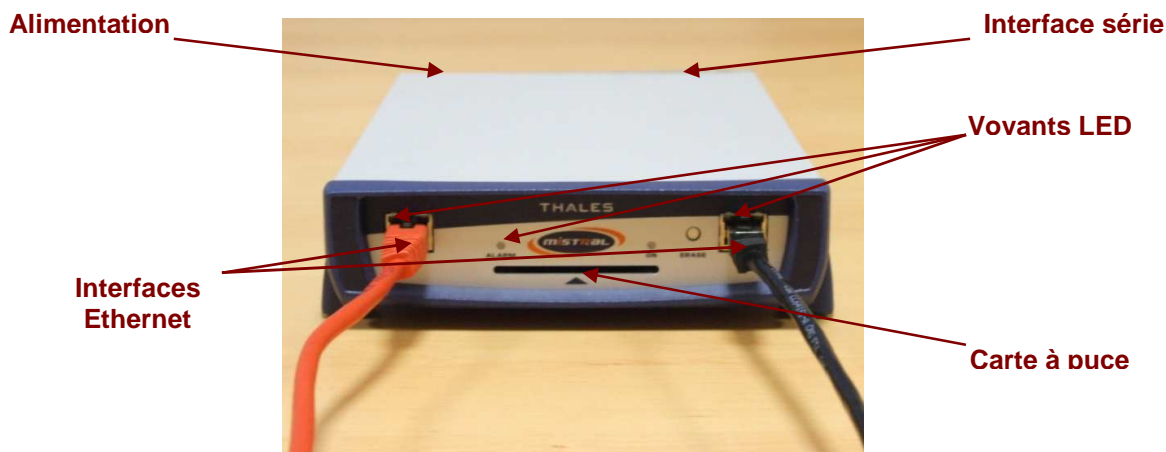
Figure 5 : Schéma des interfaces du TRC7535
